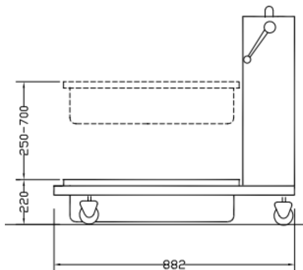
Zij aanzicht
