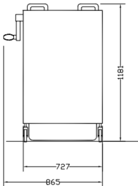
Front aanzicht
